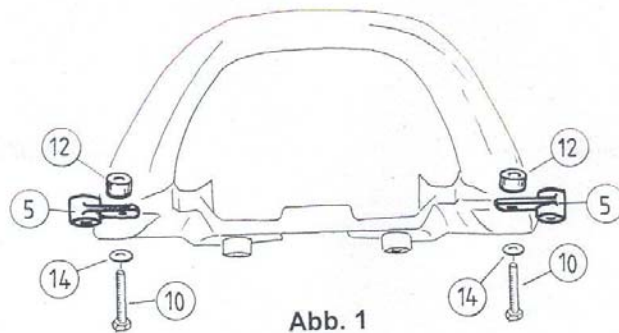
Montage der Adapterlaschen am Haltebügel
