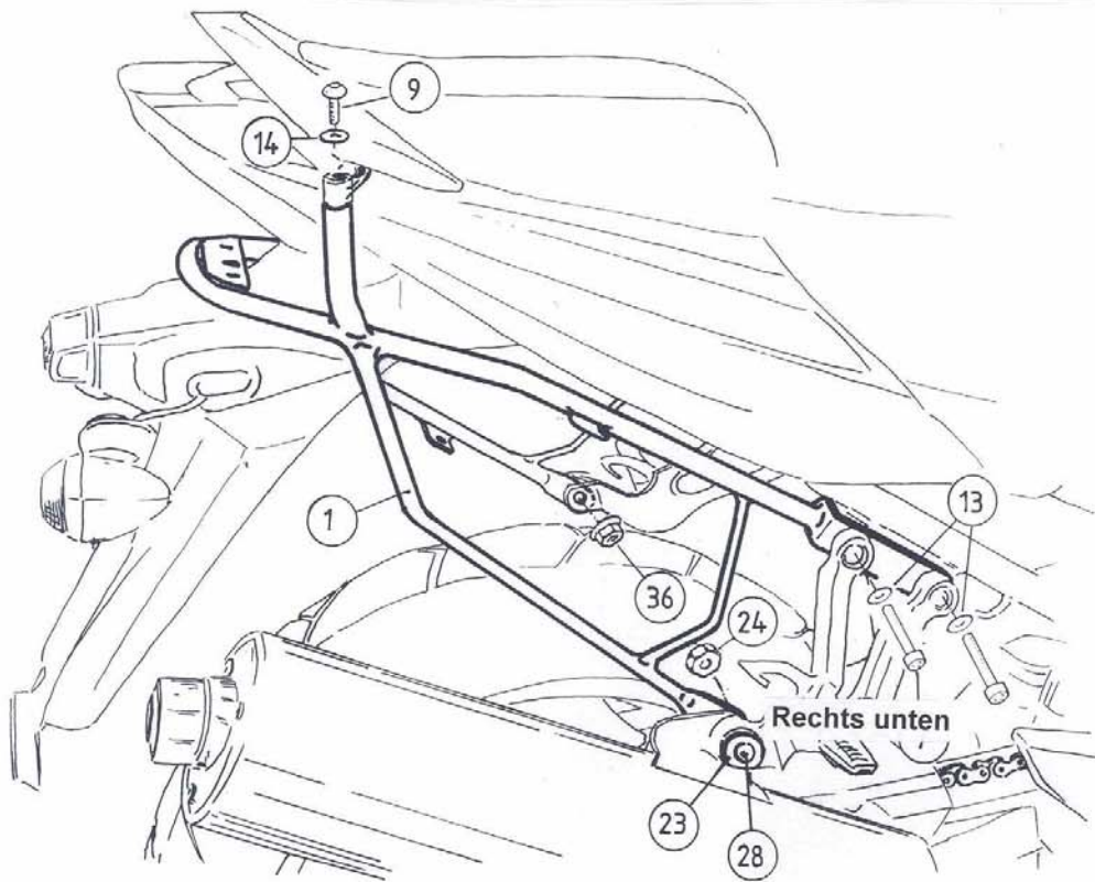
Montage des Grundrahmens (Abb. 2)
